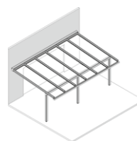
Ü3 wie Ü1, mit 3. Pfosten as Ü1, with 3 rd post
