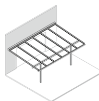
Ü2 Sparrenüberstand, Pfosten eingerrückt Purlin overhang, posts recessed
